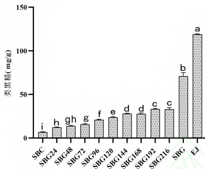
图 6 SBG、SBG 分段样品、SBC 及 EJ 的类黑精含量结果图
