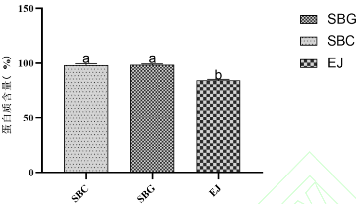
图 1 SBC、SBG 和 EJ 的总蛋白含量 Fig. 1 Total protein content of SBC, SBG, and EJ. 注: 图中不同字母表示组间差异显著 ( P<0.05 )
