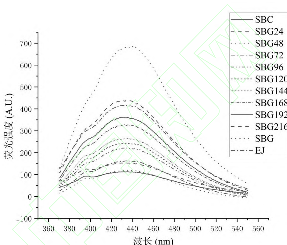
图 4 SBG、SBG 分段样品、SBC 及 EJ 的美拉德荧光产物测定结果图
