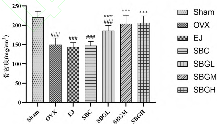
图 7 各组小鼠股骨骨密度定量分析结果
