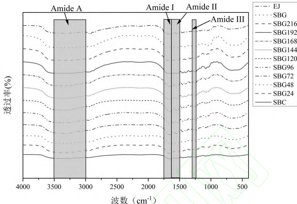
图 3 SBG、SBG 分段样品、SBC 及 EJ 的傅里叶变换红外光谱结果图 Fig. 3 Fourier transform infrared spectra of SBG, time-segmented samples of SBG, SBC, and EJ
