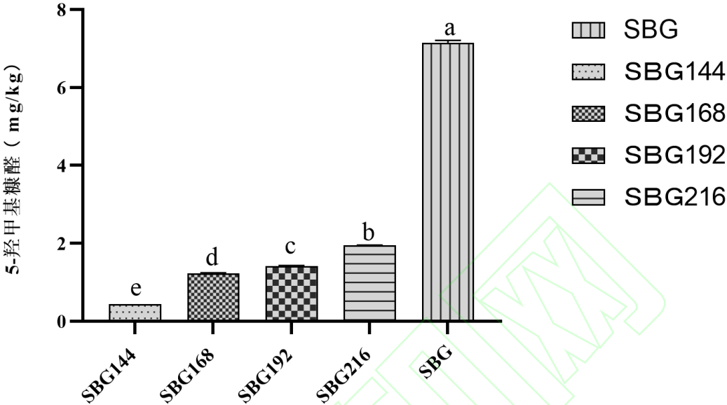
图 5 SBG 和 SBG 分段样品的 5-HMF 测定结果图
